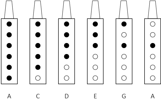
High A Pentatonic minor scale:
